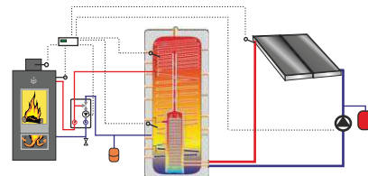
Temp. Differenzregelung Ofen mit Alarmfunktion und Temp. Differenzregelung Solar
