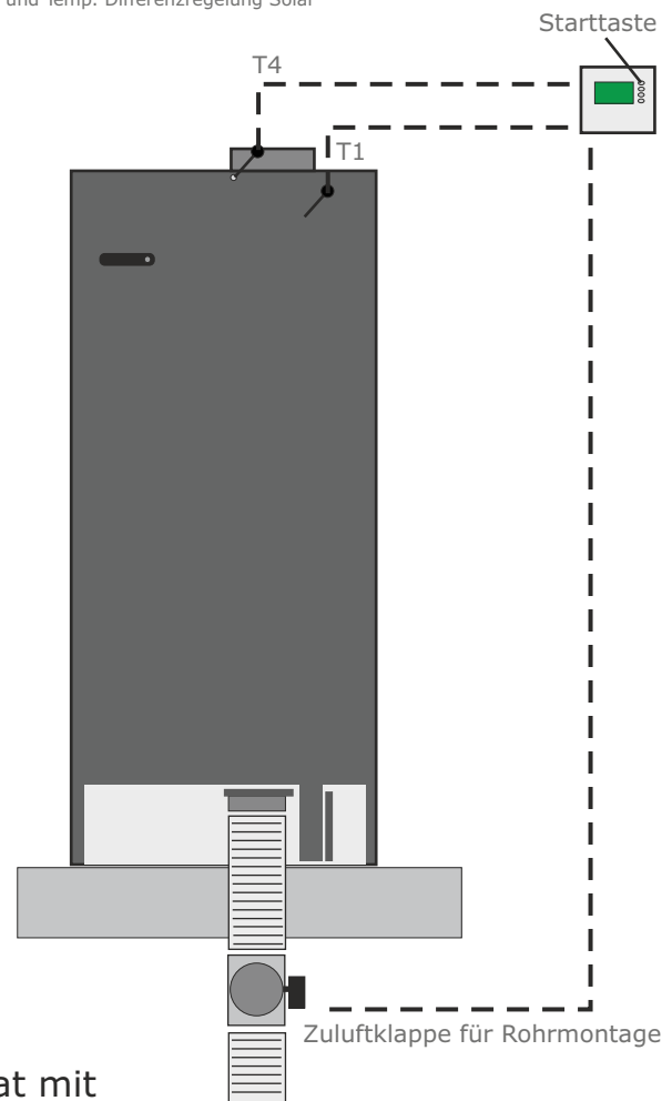
Temp. Differenzregelung Ofen mit Alarmfunktion und Temp. Differenzregelung Solar
