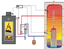
Temp. Differenzregelung Ofen + Alarmfunktion
